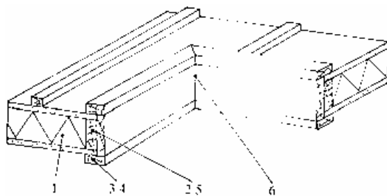
Figure 12 – Trémie avec cadre raidisseur pour fenêtre rampante
