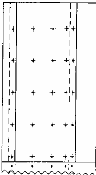
Figure 16 – Fixations des plaques FLEXOUTUILE par pointes PTM (exemple 5 fixations par rangées)
