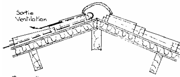
Figure 20 – Couverture en feuilles et bandes métalliques
