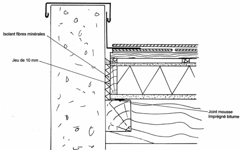
Figure 7 – Détail de rive latérale contre mur
