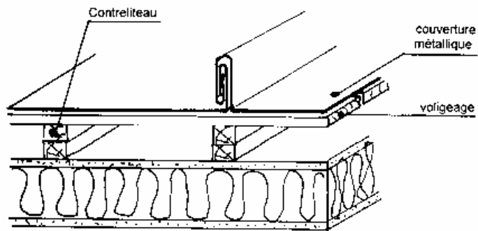
Figure 20 – Couverture en feuilles et bandes métalliques
