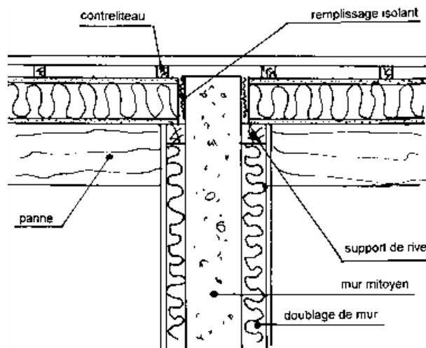
Figure 14 – Traitement acoustique de logements juxtaposés – Principe de raccordement sur refend
