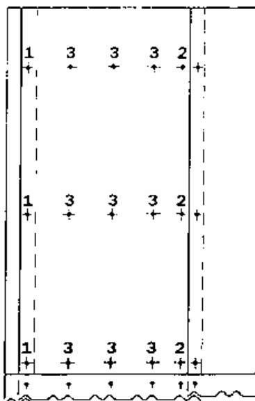
Figure 17 – Fixations des plaques FLEXOUTUILE par vis VTM
